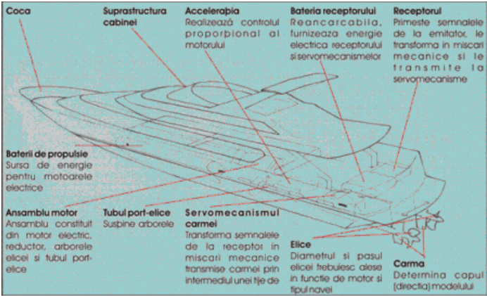
yacht cu motor (schita)
